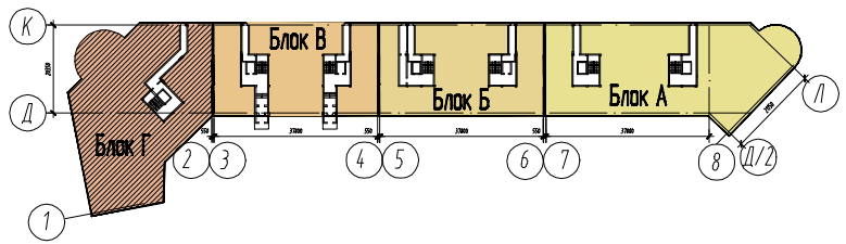
Схема блокировки
